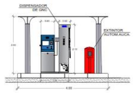
DETALLE DE IMPLANTACIÓN - ISLETAS DE DISPENSADORES ESCALA 1/50
